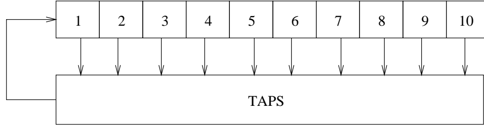
Figure 4.2. Linear Feedback Shift Register
